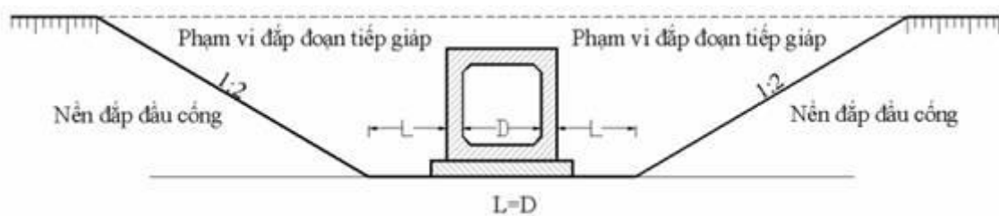
Hình 1: Phạm vi đắp đoạn tiếp giáp
